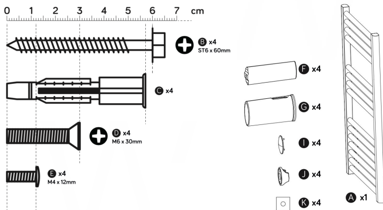
Рисунок 3. Крепежные элементы
