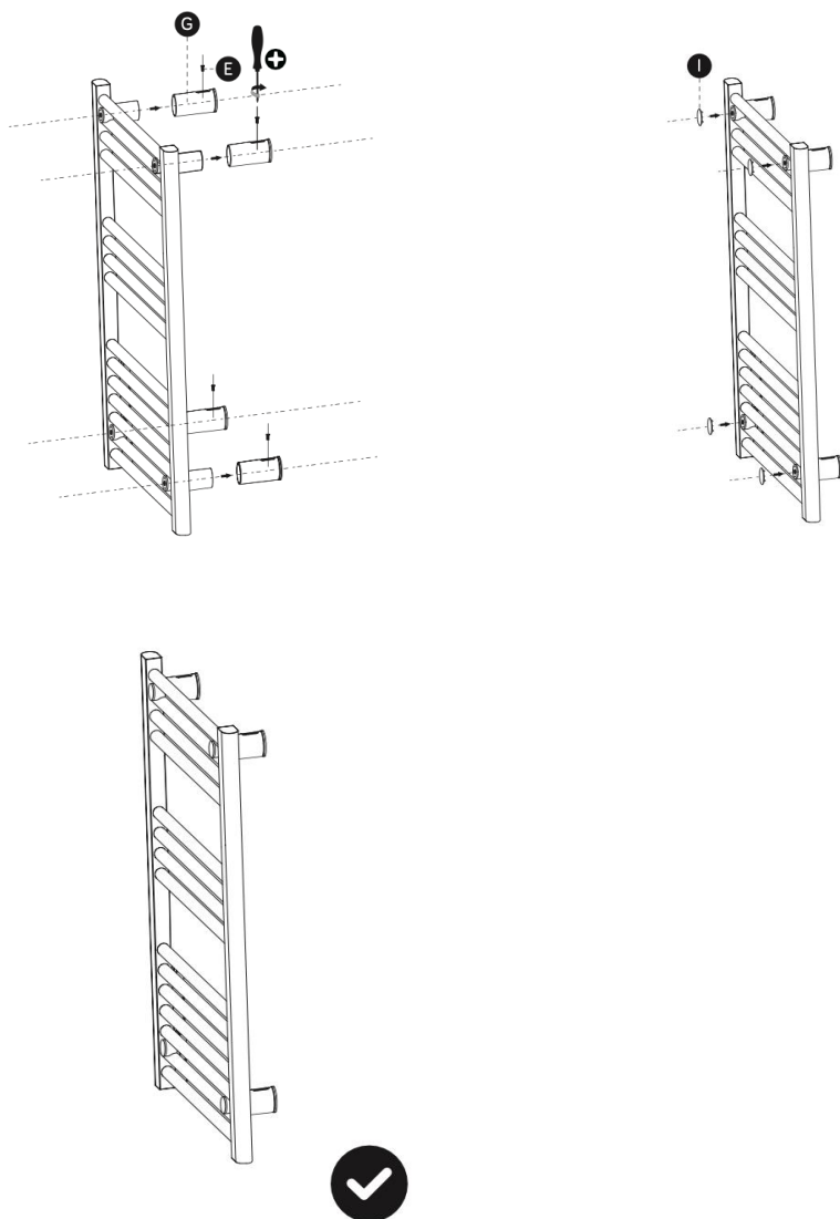
Рисунок 4. Монтаж техники
