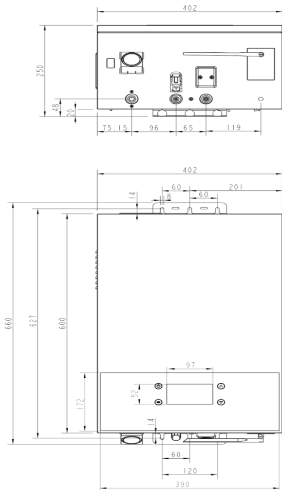
Рис.2. Габаритные размеры
