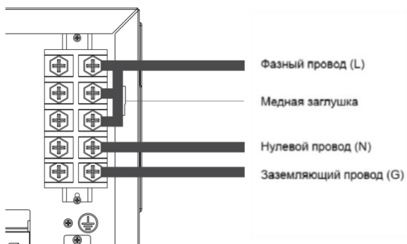
Рис. 10. Однофазное подключение прибора
