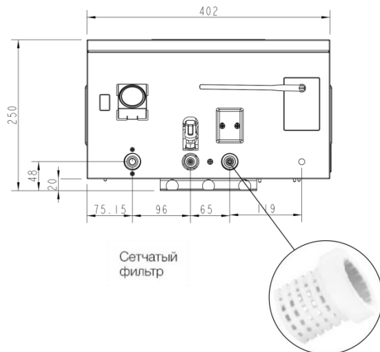
Рис. 19. Сетчатый фильтр
