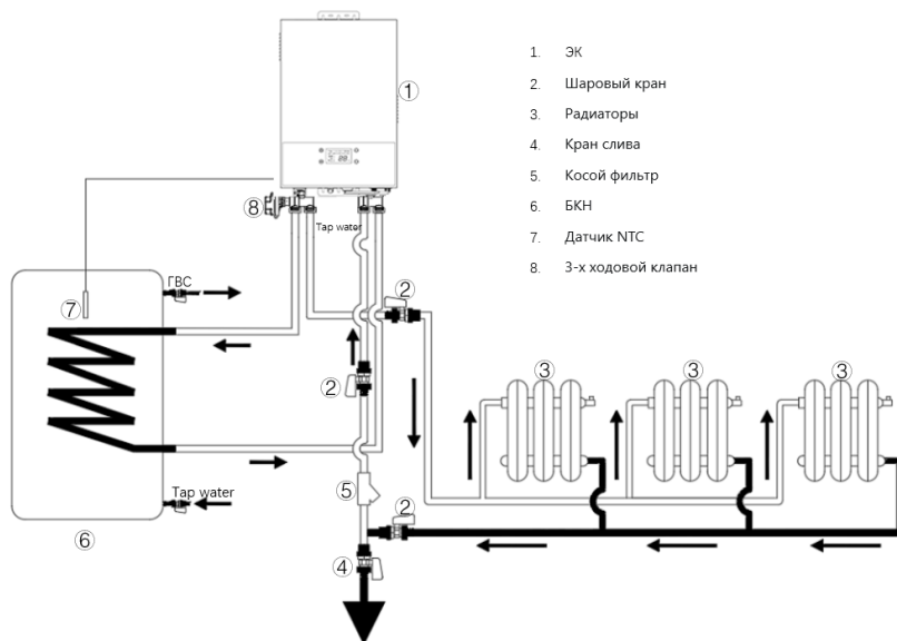
Рис. 15 Схема подключения «ЭК + БКН + радиаторы»
