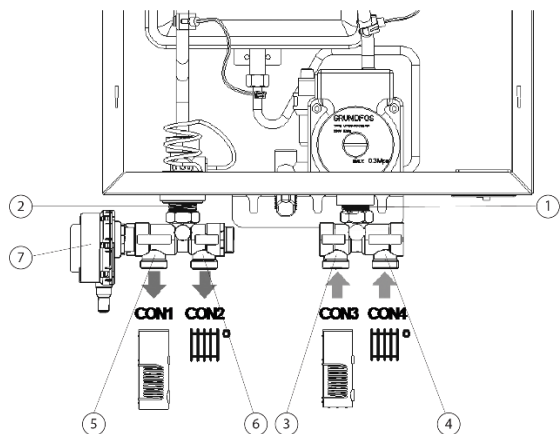
Рис.14. Схема подключения трехходового клапана
