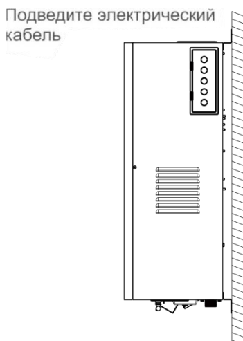
Рис. 9. Расположение панели вывода электрического кабеля
