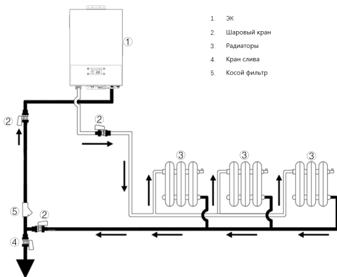
Рис. 5. Схема подключения «радиаторы + ЭК».
