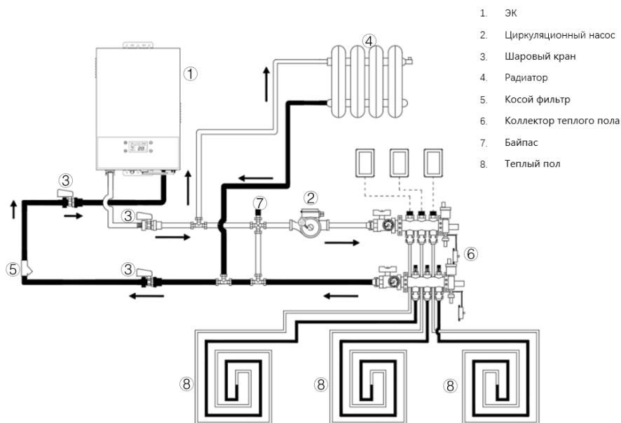
Рис. 7. Схема подключения «радиаторы + теплый пол + ЭК»
