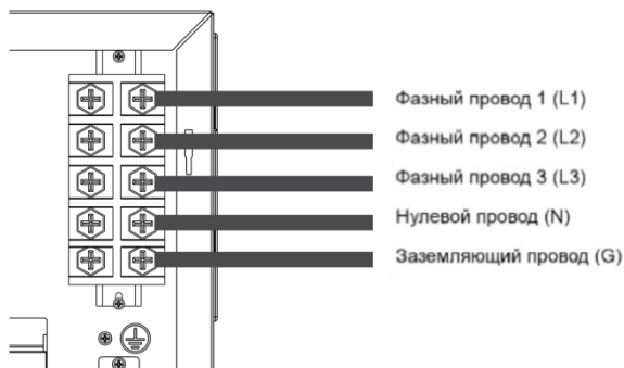
Рис. 11. Трехфазное подключение прибора
