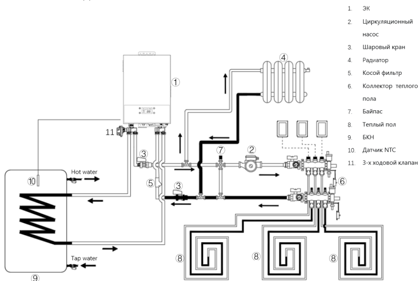
Рис. 16 Схема подключения «ЭК + БКН + теплый пол»
