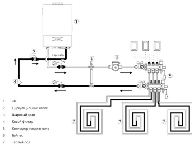
Рис. 6. Схема подключения «теплый пол + ЭК»
