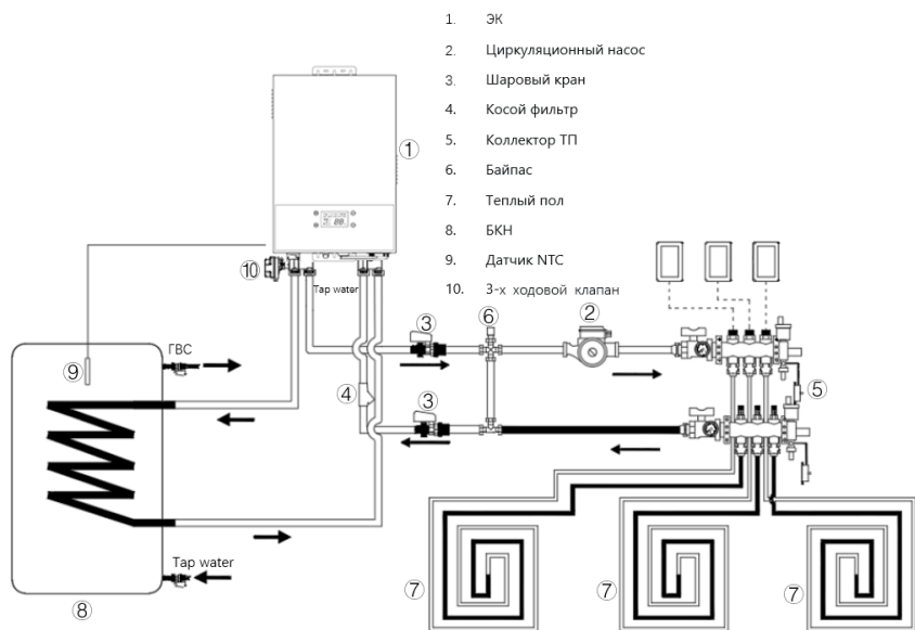
Рис. 16 Схема подключения «ЭК + БКН + теплый пол»
