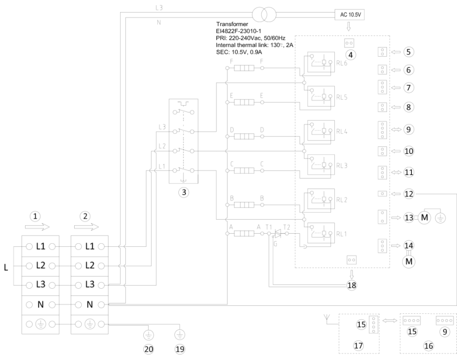
Рис. 13. Электрическая схема подключения контактов к плате управления РСВ
